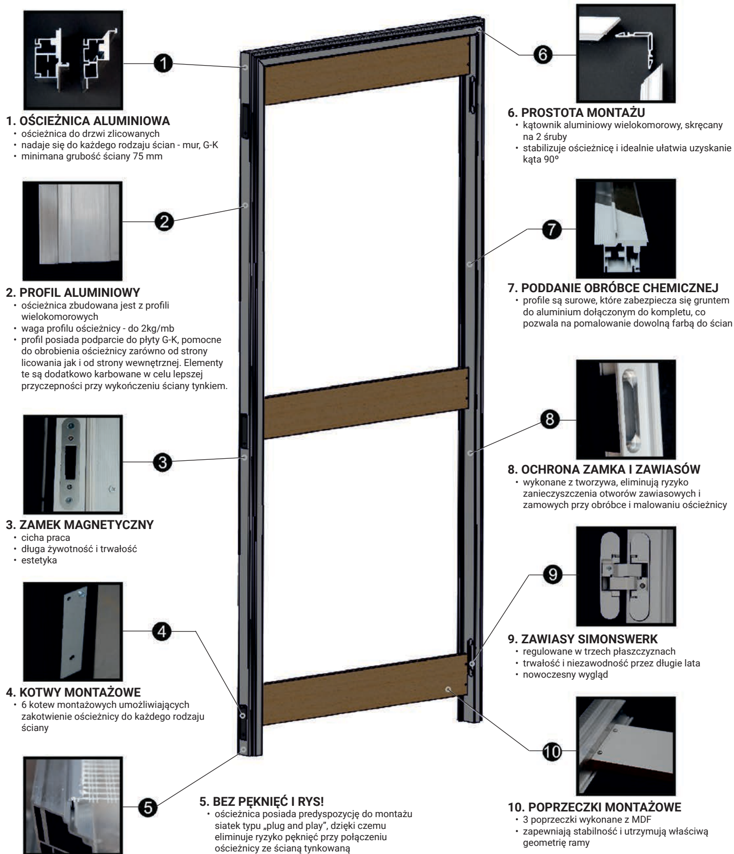
Rys. 3 – ELEMENTY KOMPLETU OŚCIEŻNICY PIU 4.2
