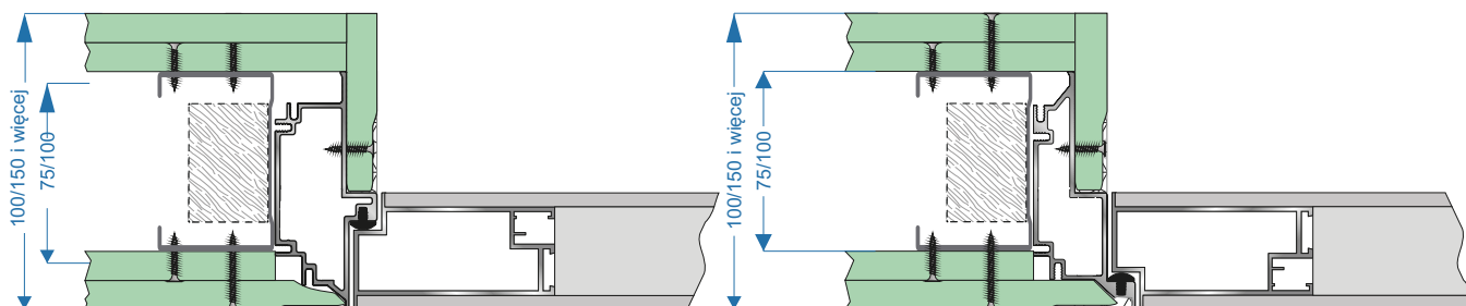
Rys. 6 – MONTAŻ OŚCIEŻNICY PIU W ŚCIANIE G-K
