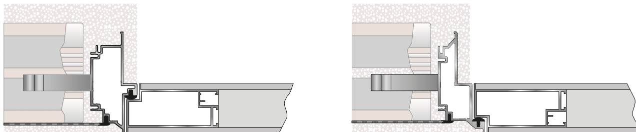
Rys. 7 – MONTAŻ OŚCIEŻNICY PIU W ŚCIANIE MUROWANEJ
