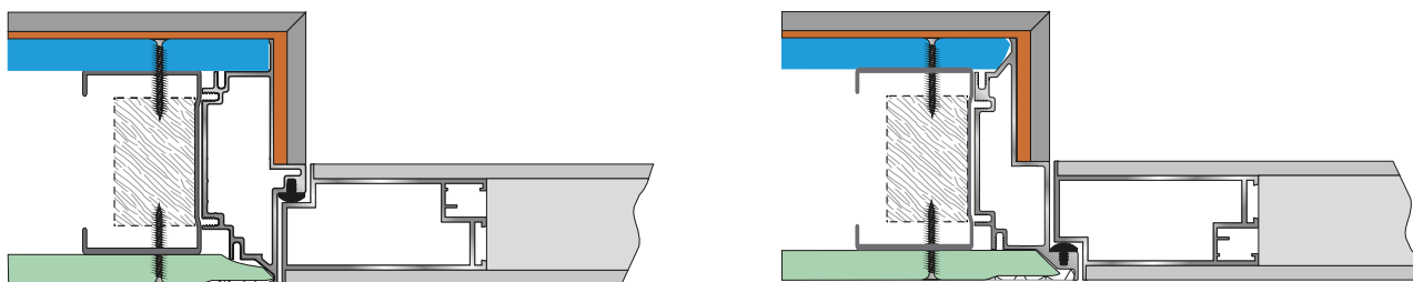
Rys. 8 – OBRÓBKA OŚCIEŻNICY PIU PŁYTKĄ CERAMICZNĄ
