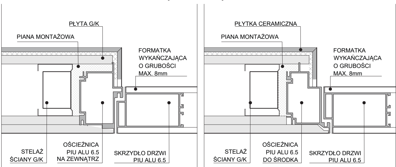
Rys. 7 – OBRÓBKA OŚCIEŻNICY PIU 6.5 Z PŁYTKĄ CERAMICZNĄ
