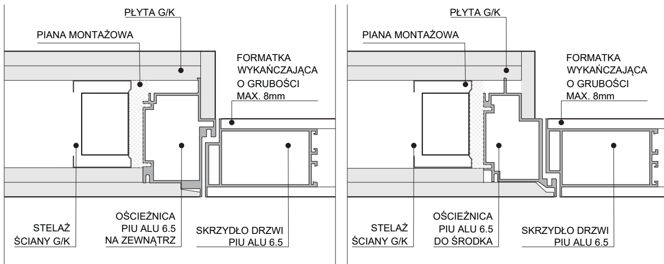
Rys. 5 – MONTAŻ OŚCIEŻNICY PIU 6.5 W ŚCIANIE G-K
