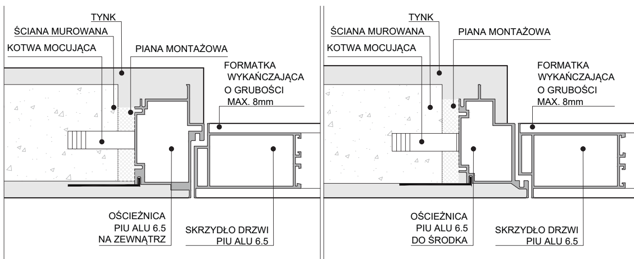
Rys. 6 – MONTAŻ OŚCIEŻNICY PIU 6.5 W ŚCIANIE MUROWANEJ
