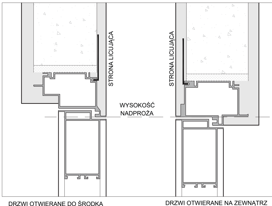
Rys. 3 – SCHEMAT RÓŻNICY WYSOKOŚCI OŚCIEŻNICY PIU TYP A I TYP B
